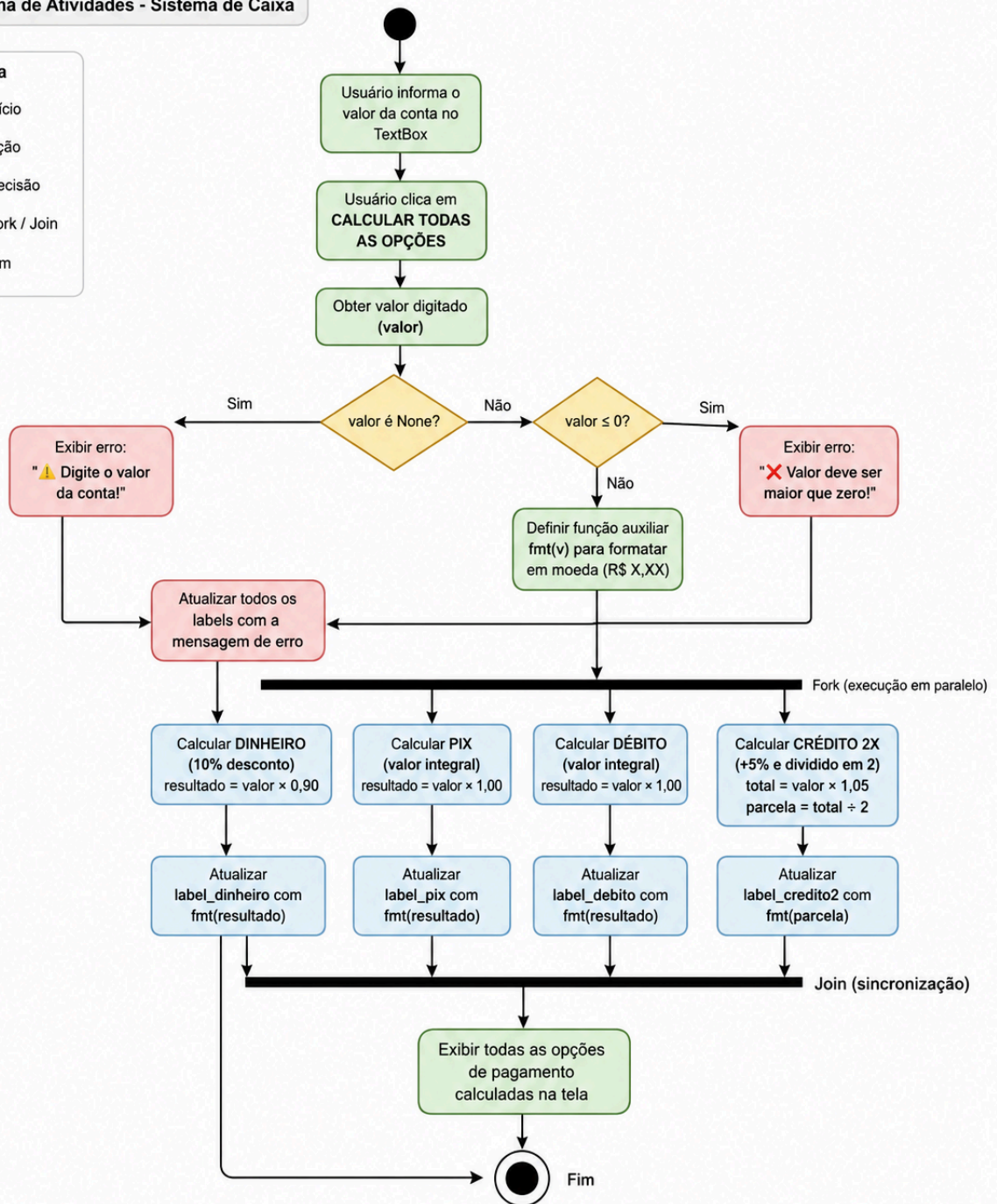
Diagrama de Atividades - Sistema de Caixa
